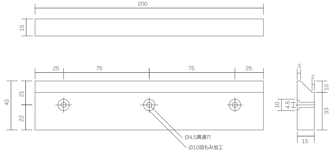
ドック形状
